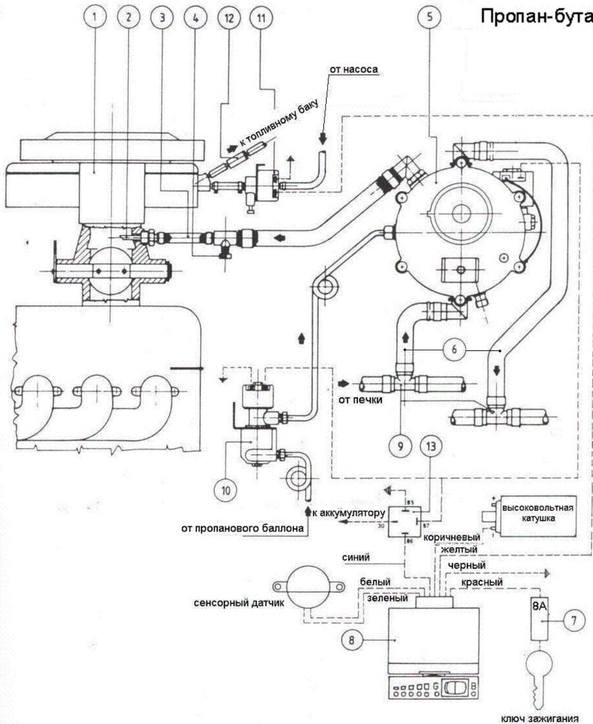
Схема подключения электронного редуктора М84 на автомобиль с карбюратором
