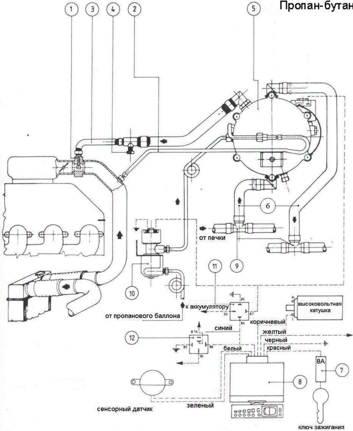
Схема подключения электронного редуктора M84 Turbo на автомобиль с Turbo инжектором
