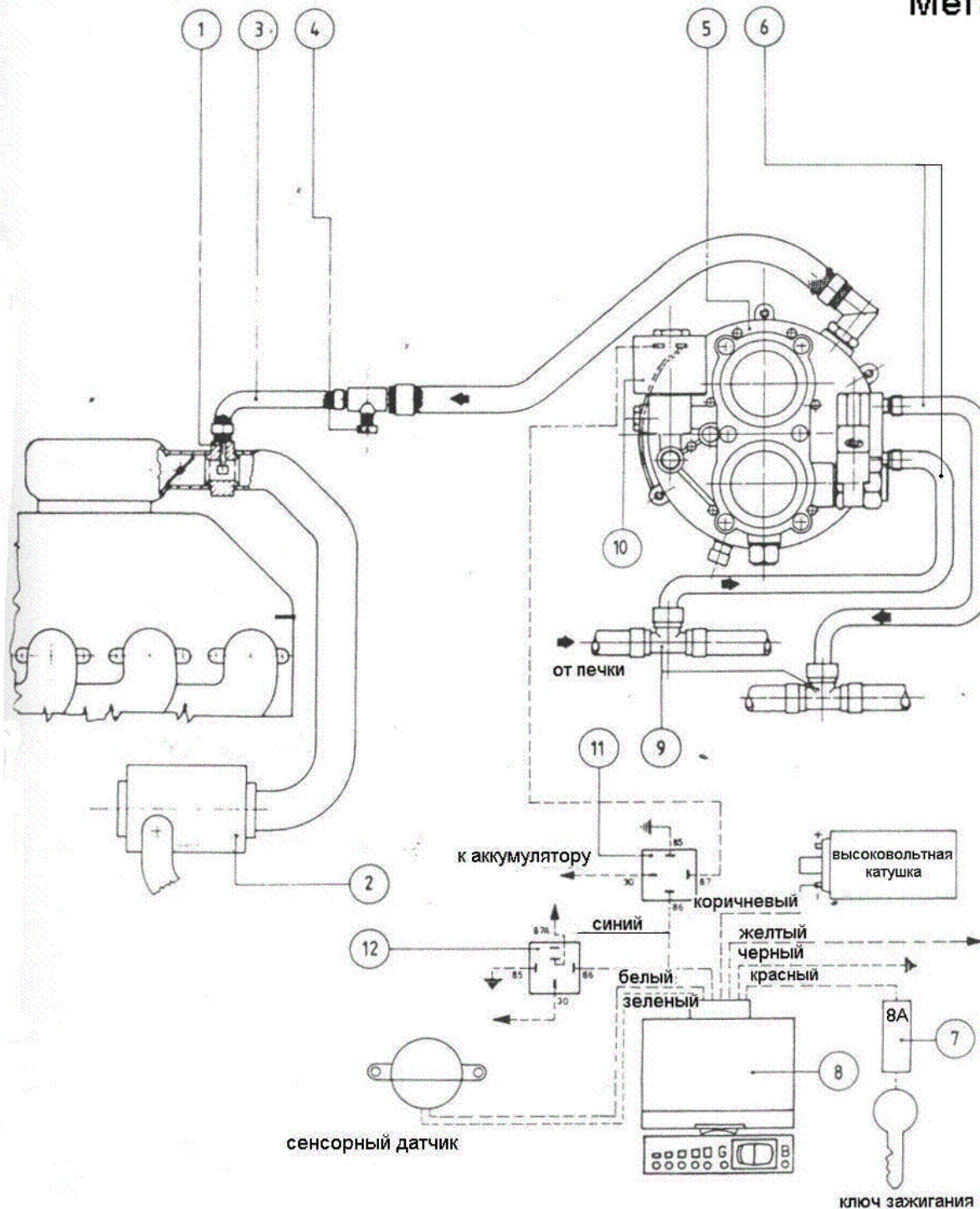
Схема подключения электронного редуктора М96/97 на автомобиль с инжектором
