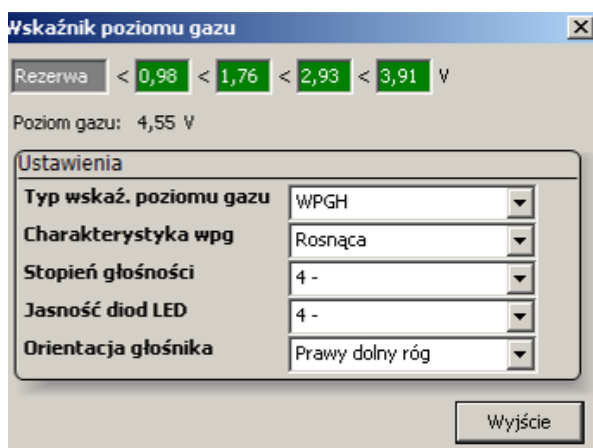
Рис. 2.3.2 Окно конфигурации LED-400
