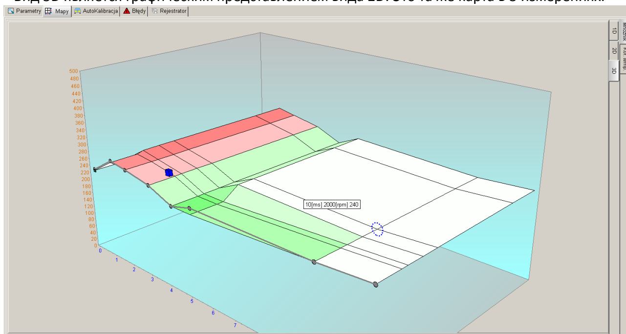
Рис. 2.1.13 Карта 3D.
