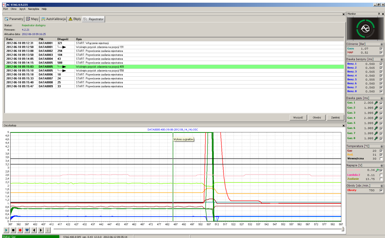
Рис. 2.1.19 Окно «Регистратор».
