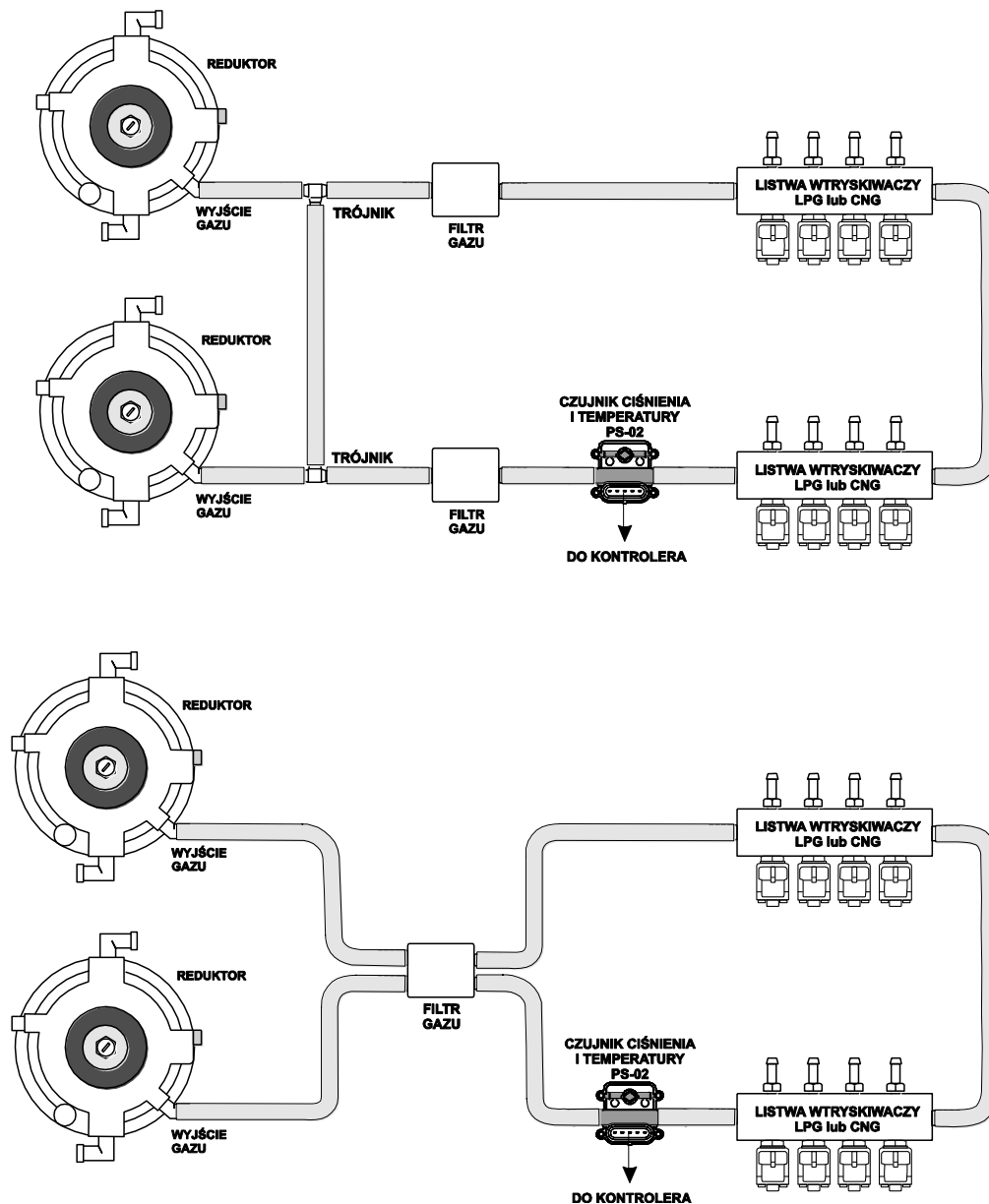
Рис. 1.3.29 Рекомендуемые схемы подключения двух редукторов.
