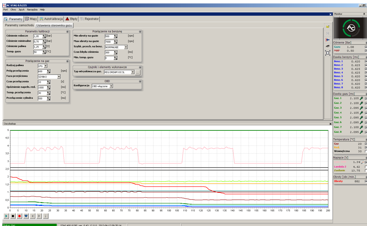
Рис. 2.1.2а Окно «Параметры» (Настройки контроллера газа).
